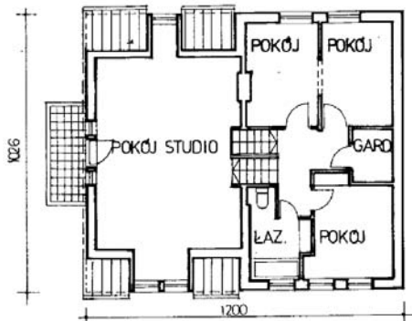
RZUT PIĘTRA
