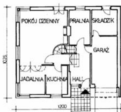
RZUT PARTERU
