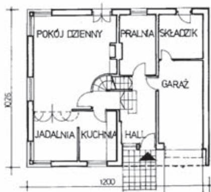
RZUT PARTERU
