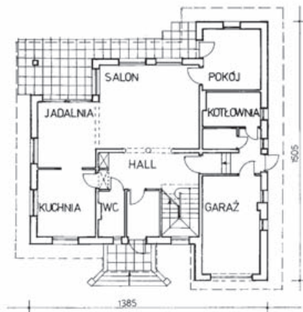
RZUT PARTERU
